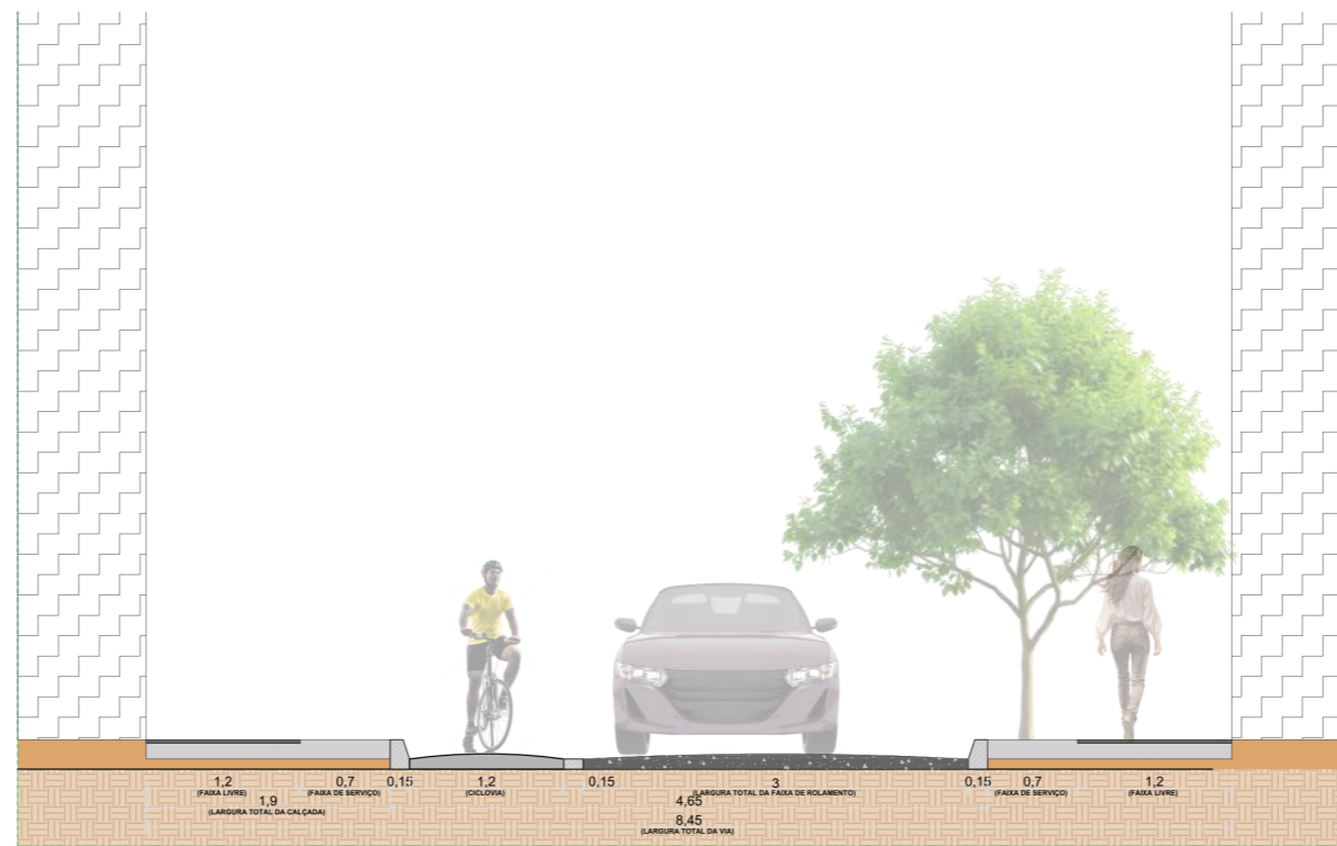
ESCALA 1:20 VIA COMPLETA - LOCAL
