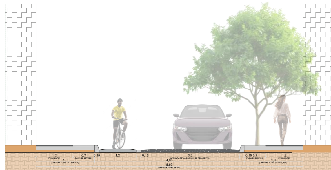
ESCALA 1:20 VIA COMPLETA - COLETORA
