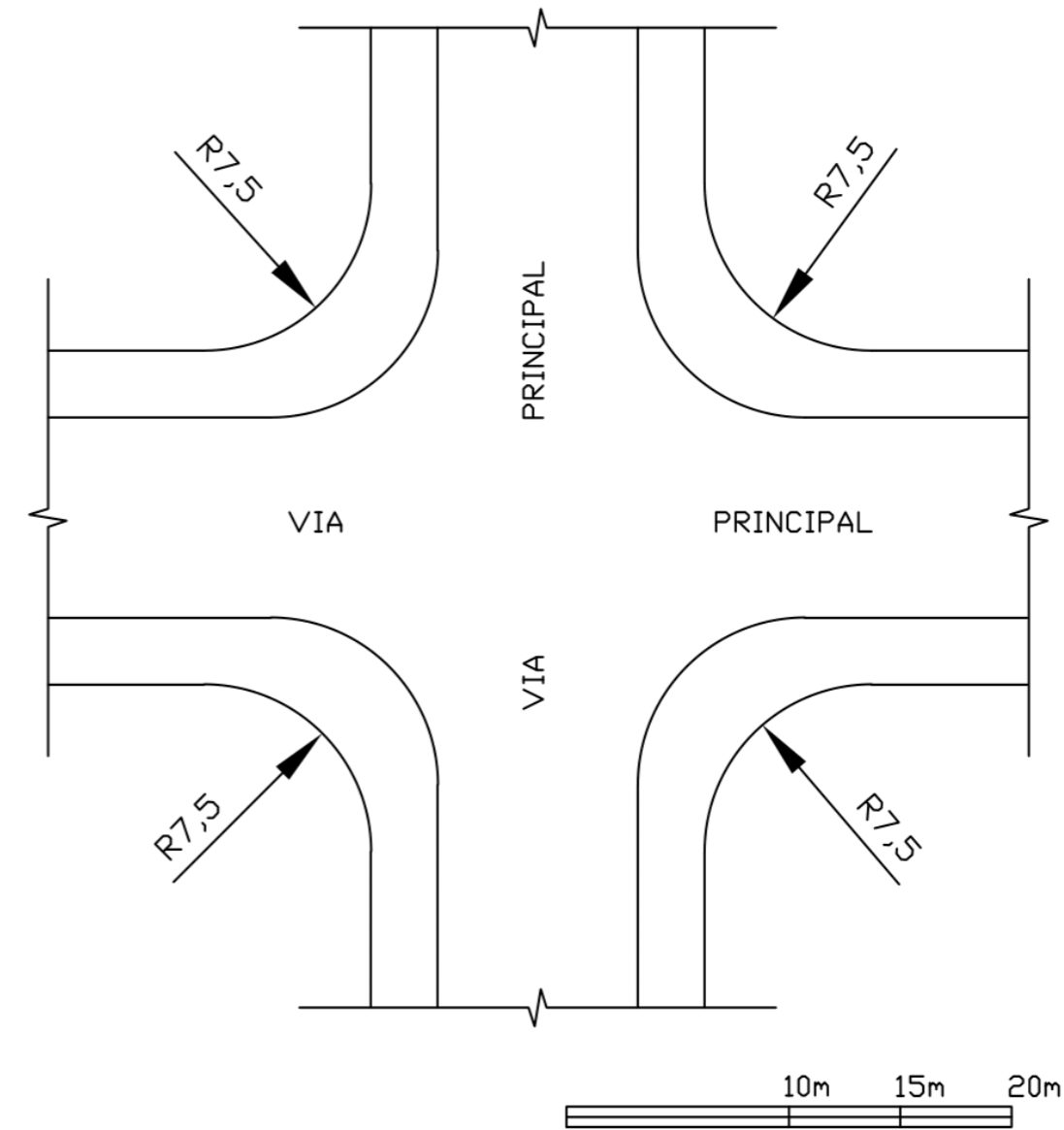
CRUZAMENTO COLETORA COLETORA X COLETORA
